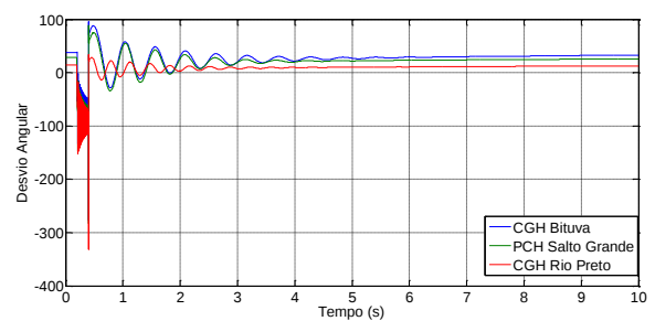
Figura 7 – Curto-circuito na subestação no instante t=0,2s . Com os controladores PSS.
