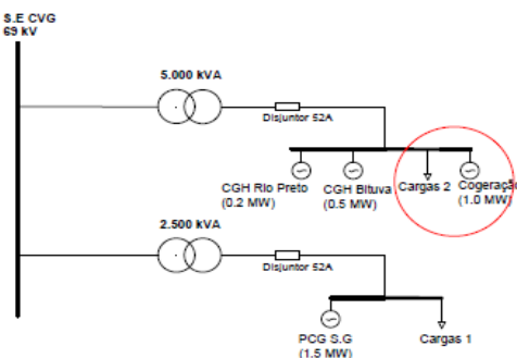
Figura 3 – Sistema de Distribuição da Empresa CVG. Considerando a inclusão do sistema de cogeração.
