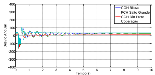
Figura 8 - Curto-circuito na subestação no instante t=0,2s , com o sistema de cogeração
