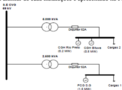
Figura 1- Sistema de Distribuição da Empresa CVG.
