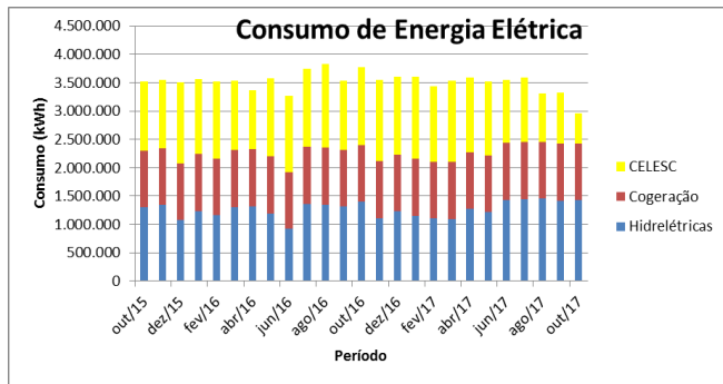
Figura 4 – Consumo de energia elétrica com a participação do sistema de cogeração.
