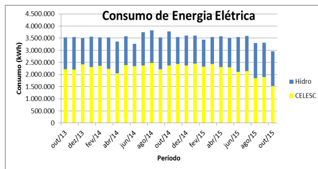
Figura 2 - Histórico do consumo de energia elétrica.
