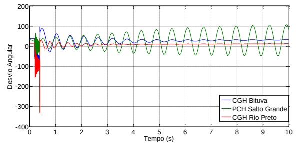
Figura 6 – Curto-circuito na subestação no instante t=0,2s . Sem os controladores PSS.
