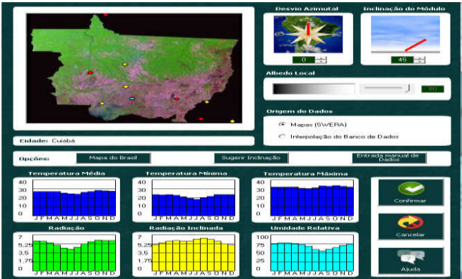
Figura 7. Estimativa Radiação local (Fonte: RadiaSol2)
