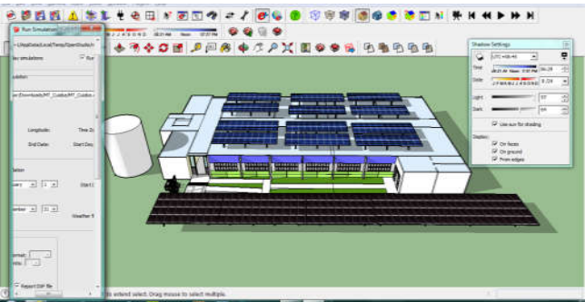
Figura 5 Modelagem da planta do Bloco C.
