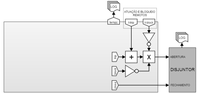
Figura 1. Estrutura computacional base do relé
