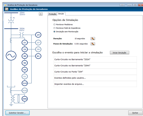
Figura 9. Tela inicial da simulação do defeito na barra 138kV da unidade A de Fontes Nova
