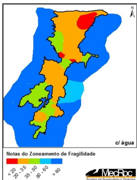
Figura 5. Resultado do zoneamento geotécnico da cavidade CAI-03 simulada para o maciço com água.
