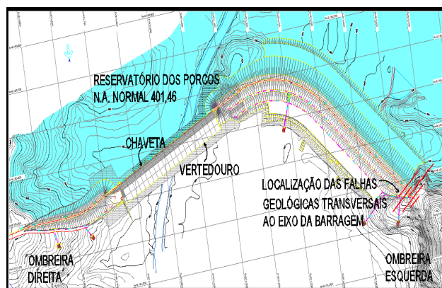
Figura 2. Planta de Arranjo Geral do Projeto da Barragem de Porcos. Modificado de Consórcio Hidroconsult-MWH do Brasil (2012). Planta1220-DES-1113-20-15-001. R04.
