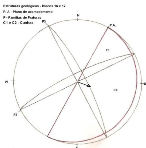
Figura 8. Estruturas geológicas identificadas na fundação do vertedouro nos blocos 16 e 17. A seta indica a direção do mergulho principal de acamamento e em C1 e C2 a visualização das cunhas de ruptura.
