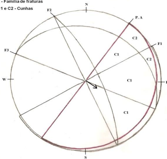
Figura 4. Estruturas geológicas identificadas na fundação do vertedouro nos blocos 13, 14 e 15 lançadas em rede estereográfica de Schmidt.
