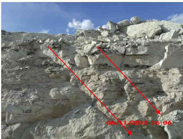
Figura 5. Sistema de fraturas considerado crítico para a barragem, família F3 encontrada nas camadas de siltito com penetração nas camadas de arenito.
