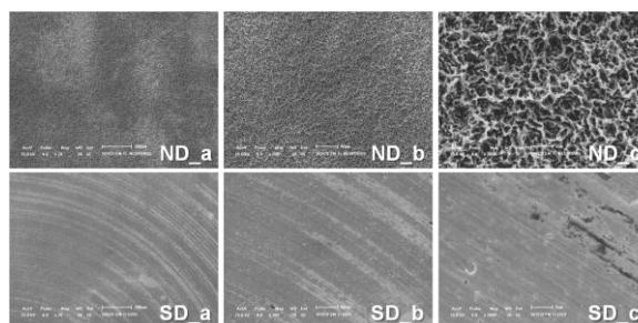
Figura 4: MEV dos discos de titânio – Disco Neoporos (DN) e Disco Usinado (DU) com ampliações de 70x (a), 200x (b), 2000x (c).
