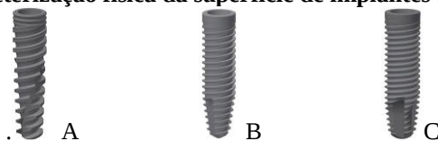
Figura 1: Macrogeometrias dos Implantes. A – Drive; B – Alvim; C – Titamax EX
