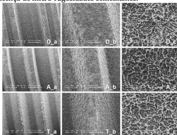
Figura 3: MEV dos implantes - Drive (D), Alvim (A) e Titamax EX (T) em ampliações de 70x (a), 200x (b), 2000x (c).
