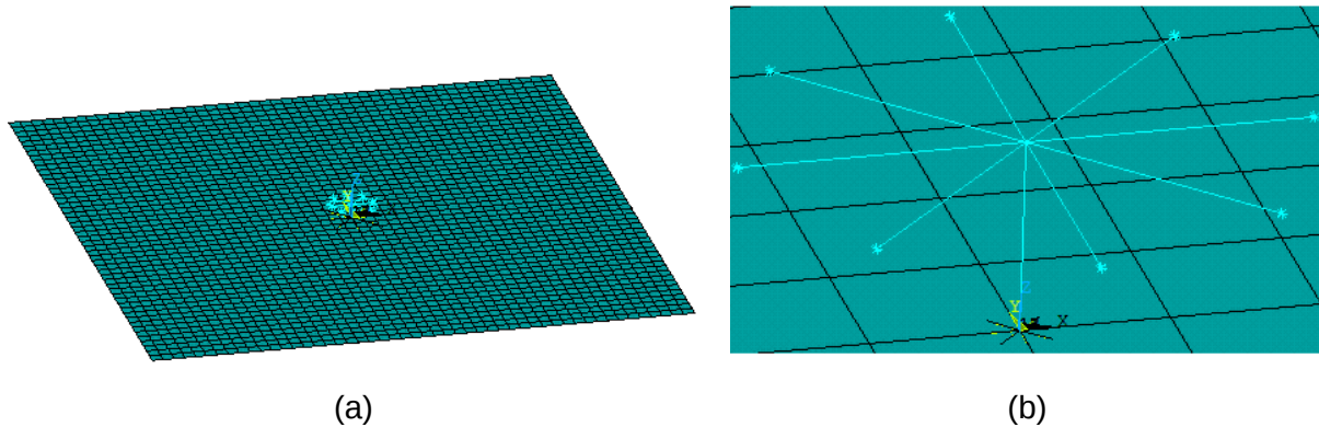
Figura 2: a) estrutura acoplada; b) detalhe do ADV
