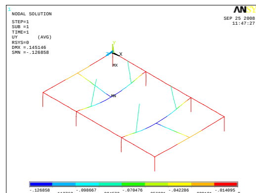
Figura 2: Visualização dos deslocamentos na direção y na estrutura.
