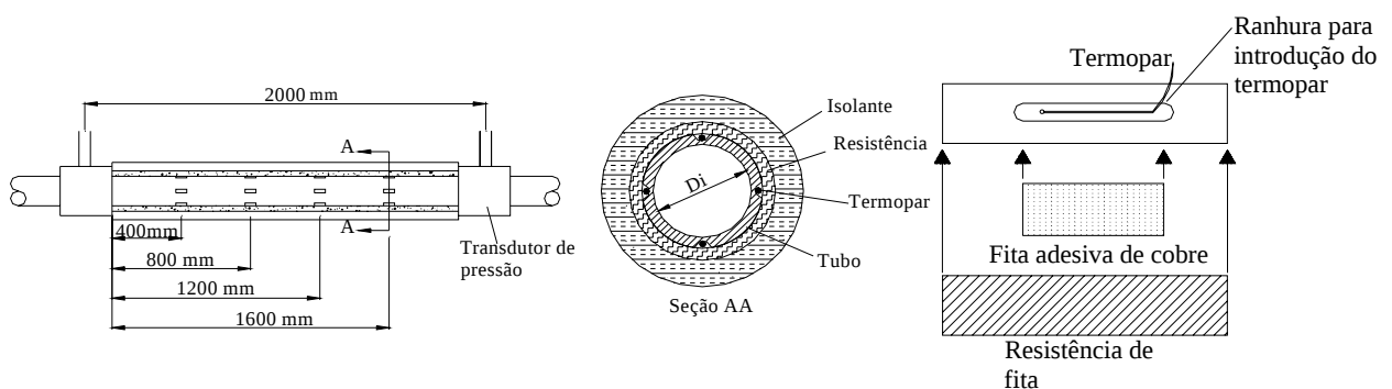
Figura 3. Detalhe da seção de testes e da instalação dos termopares de medida da temperatura superficial.
