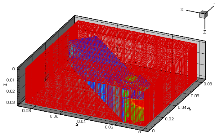
Figura 2: Visualização tridimensional do campo de temperatura obtido numericamente para o modelo proposto na Equação (1)
