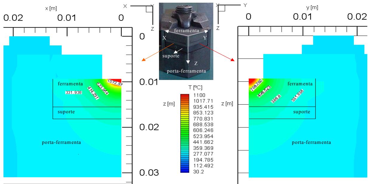
Figura 7: Vista lateral dos campos de temperatura (planos x-z e y-z) no instante t = 60 s para a condição mais severa
