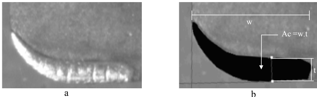
Figura 4: a) Visualização da área de contato através da câmera de vídeo e b) Tratamento da imagem realizado pelo software GLOBAL LAB Image
