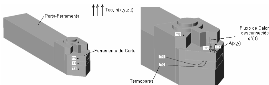
Figura 3: Posicionamento dos termopares T_1 a T_8 no conjunto ferramenta e porta-ferramenta
