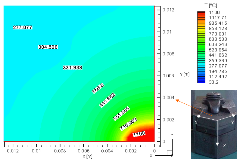
Figura 6: Vista superior do campo de temperatura (plano x-y) no instante t = 60 s para a condição mais severa
