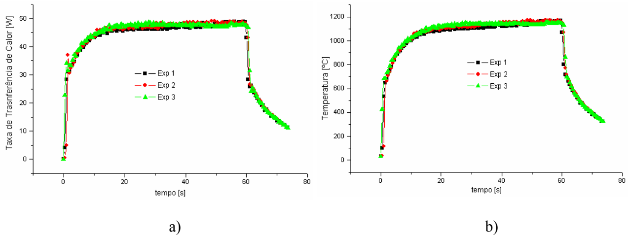
Figura 5: a) Taxa de transferência de calor estimada para a condição de usinagem mais severa de três experimentos b) Comparação entre as temperaturas estimadas para as taxas da Figura (5a)
