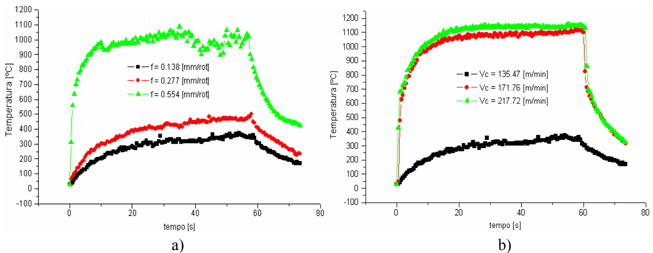
Figura 8: Temperaturas na interface cavaco-ferramenta considerando a) v_c = 135,3 m/min, a_p = 1,5 mm no raio e 3 avanços diferentes e b) 3 velocidades de corte diferentes, a_p = 1,5 mm no raio e f = 0,138 mm/rot
