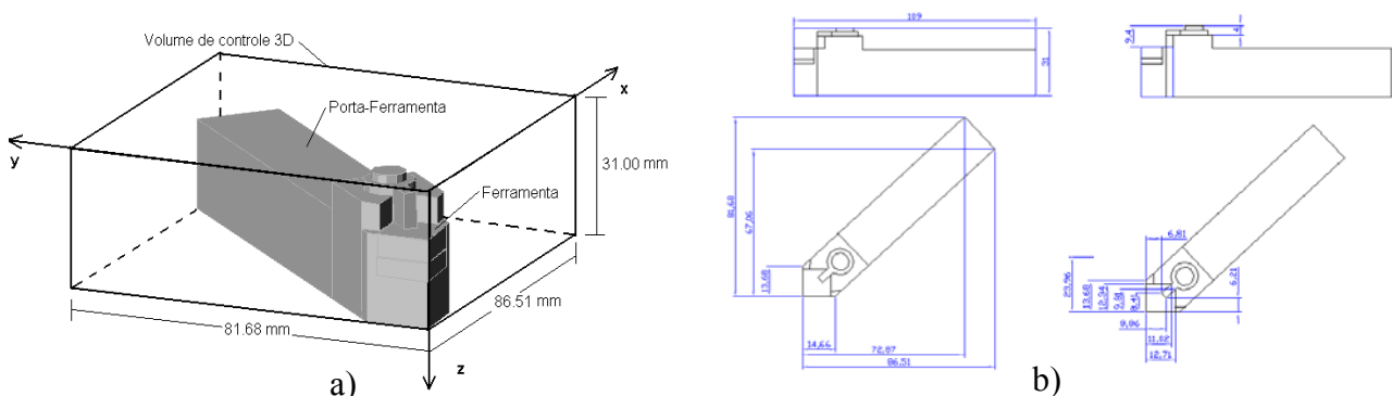
Figura 1: a) Problema térmico tridimensional da ferramenta e porta-ferramenta e b) Dimensões do conjunto ferramenta e porta ferramenta
