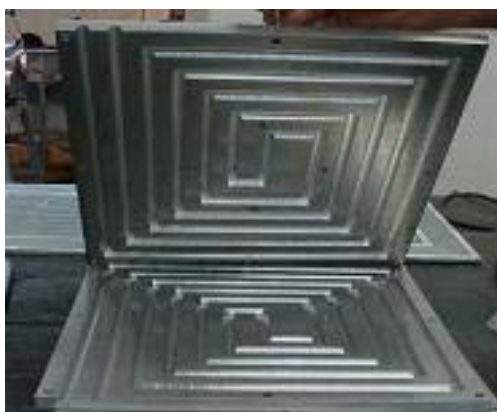
Figura 5: Placa fria depois de usinada
