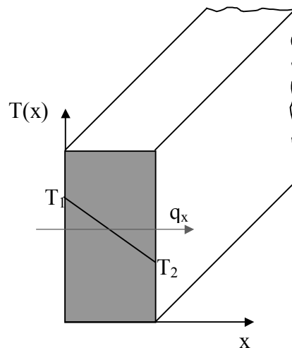
Figura 1- Campo térmico em uma parede plana com temperaturas T_1 e T_2 em suas superfícies.
