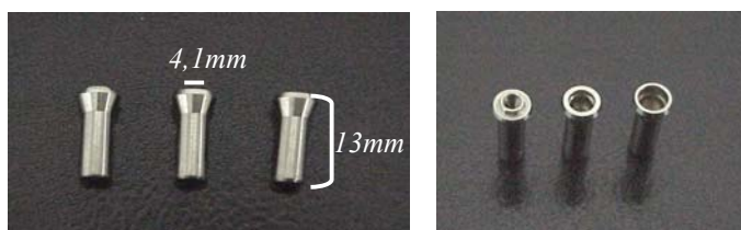
Figura 1: dimensões principais dos implantes utilizados.
