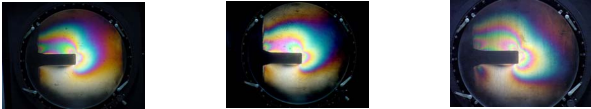
Figura 5: Distribuição das franjas para os implantes E, I e C sob carga tipo 2.
