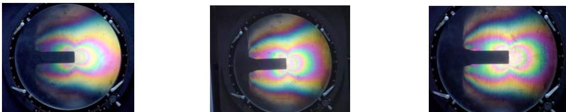
Figura 4: Distribuição das franjas para os implantes E, I e C sob carga tipo 1.
