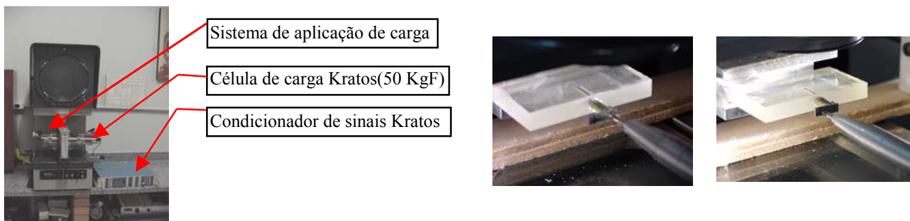
Figura 3: Esquema da montagem experimental e a carga 1 e carga 2 aplicadas no modelo fotoelástico.
