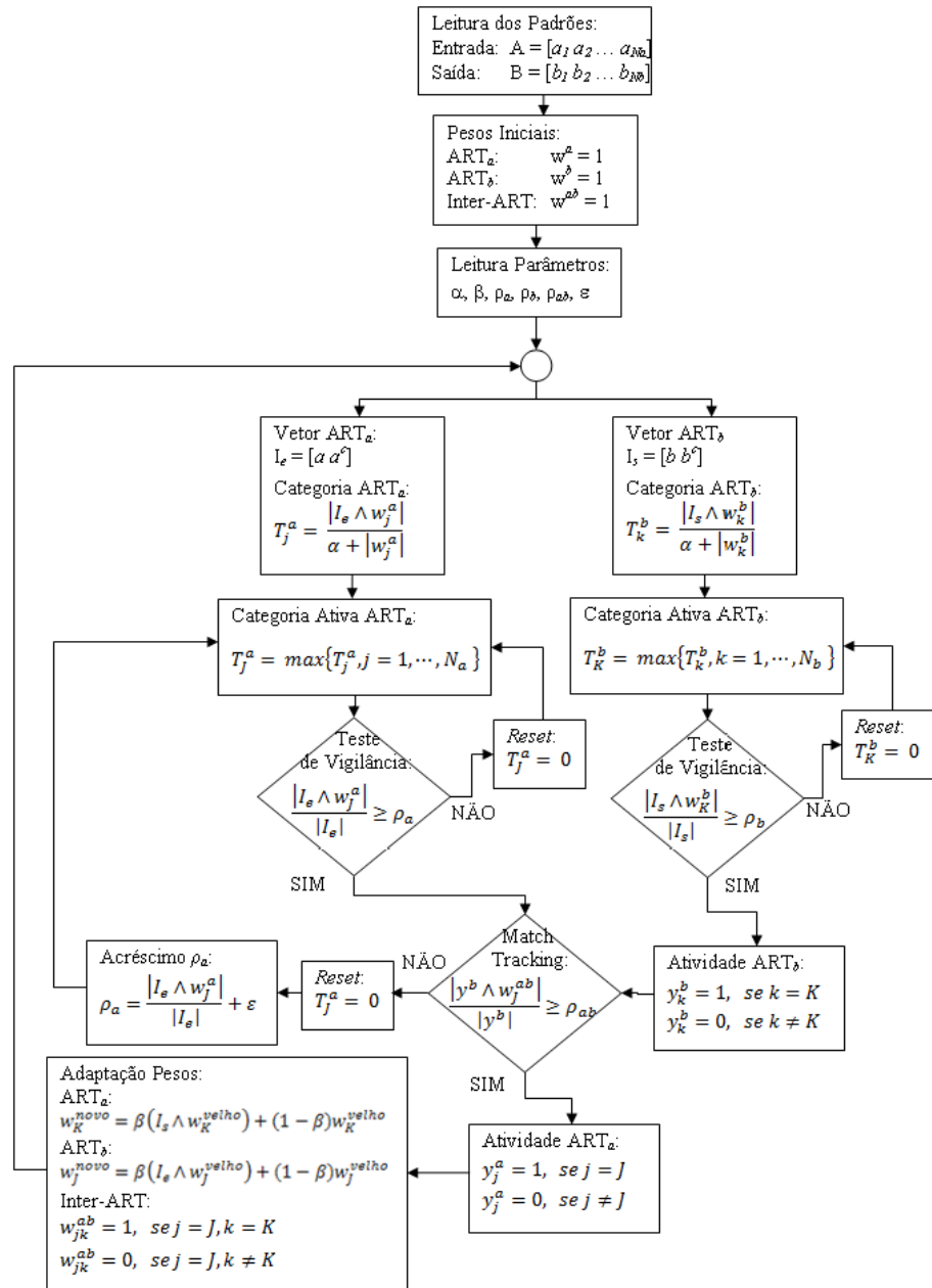
Figura 2: Fluxograma do treinamento da rede neural ARTMAP Fuzzy.
