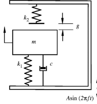
Figura 1: Modelo do sistema vibro-impacto [3].
