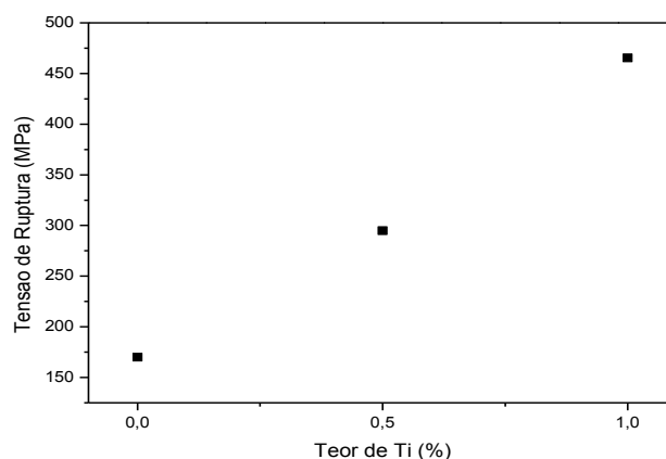
Figura 8. Gráfico Tensão de Ruptura versus Teor de Ti na liga de Cu-Al-Be (%w).
