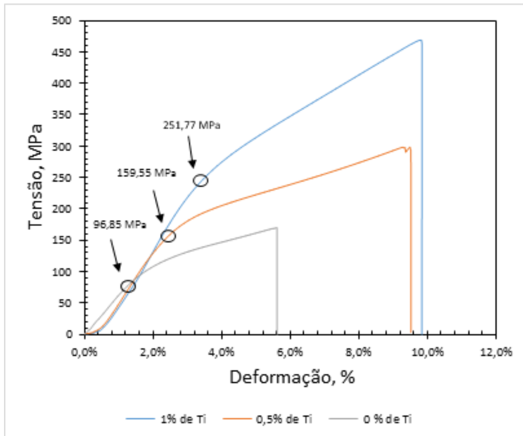
Figura 6. Ensaio de tração na liga de Cu-Al-Be com 0%, 0,5% e 1% de Ti (%w).
