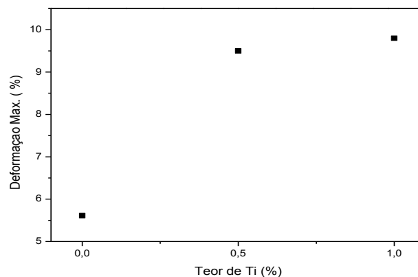
Figura 7 - Gráfico Deformação versus Teor de Ti na liga de Cu-Al-Be (%w).
