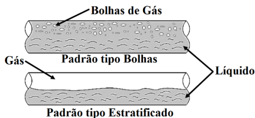
Figura 1. Padrão de escoamento tipo Bolhas e Estratificado.
