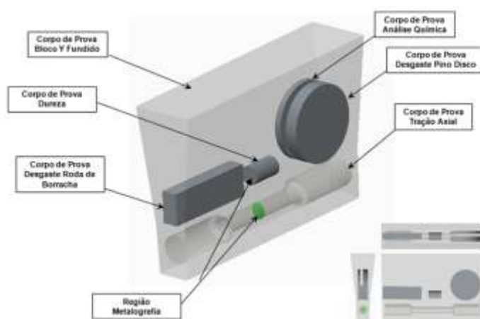
Figura 1. Corpo de prova modelo "Y".
