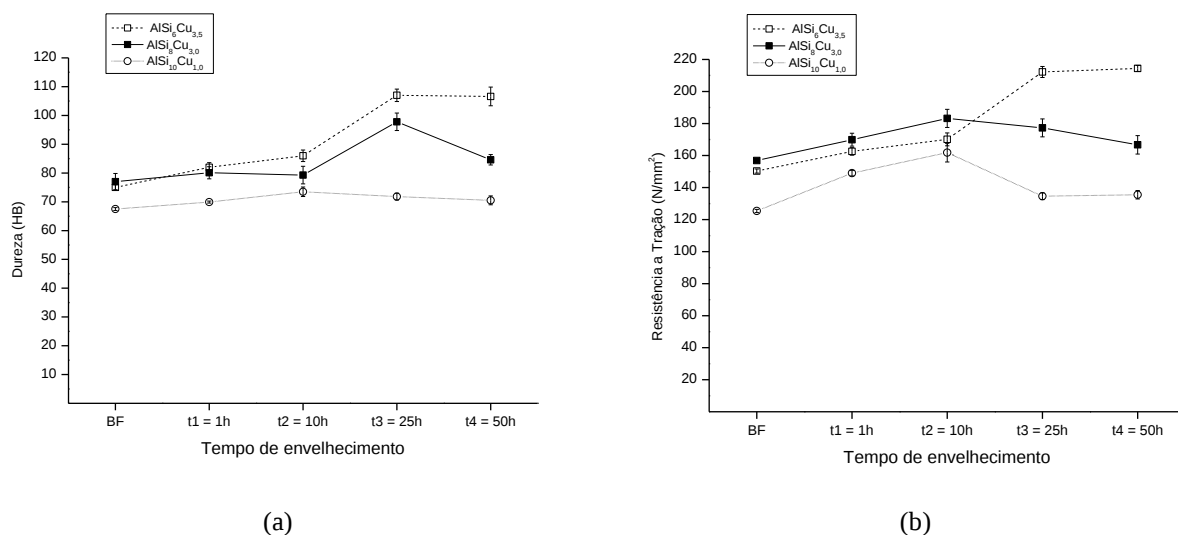
Figura 9. Dureza (a) e Resistência a tração (b) na condição após tratamento térmico.
