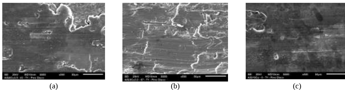
(a) (b) (c) Figura 14. Pista de desgaste das ligas \text{AlSi}_6\text{Cu}_{3,5} (a), \text{AlSi}_8\text{Cu}_{3,0} (b) e \text{AlSi}_{10}\text{Cu}_{1,0} (c) na condição bruto de fundição após ensaio de desgaste pino sobre disco, tempo 50h.
