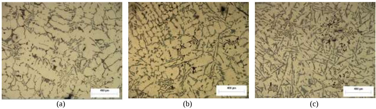
Figura 6. Microestrutura das ligas \text{AlSi}_6\text{Cu}_{3,5} (a), \text{AlSi}_8\text{Cu}_{3,0} (b) e \text{AlSi}_{10}\text{Cu}_{1,0} (c) condição bruta de fundição, ataque HF 0,5%.
