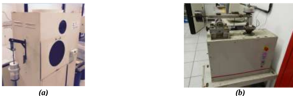
Figura 5. Abrasômetro tipo roda de borracha (a) e tribômetro pino sobre disco (b).
