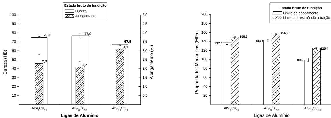
Figura 8. Dureza e alongamento (a) e resistência a tração e limite de escoamento (b) na condição de bruto de fundição.
