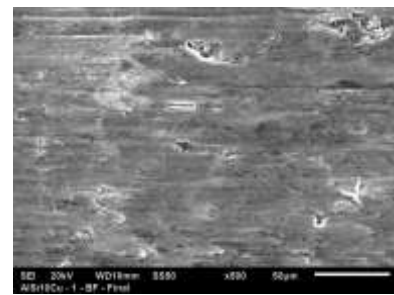
Figura 11. Pista de desgaste das ligas \text{AlSi}_6\text{Cu}_{3,5} (a), \text{AlSi}_8\text{Cu}_{3,0} (b) e \text{AlSi}_{10}\text{Cu}_{1,0} (c) na condição bruta de fundição após ensaio de desgaste roda de borracha.
