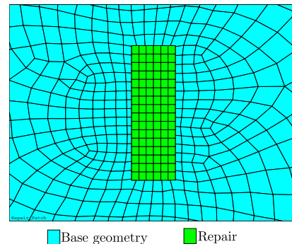
(d) Repair patch in detail, area 8.54cm 2 .
