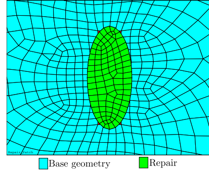
(d) Repair patch in detail, area 10.32cm 2 .
