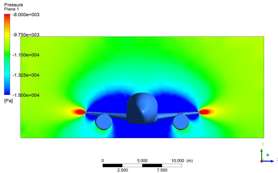
Figura 7. Plano de pressão no eixo YZ posicionado sobre as asas na velocidade máxima
