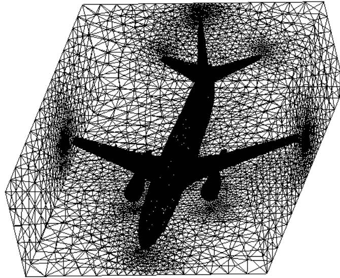
Figura 3. Malha em torno da geometria
