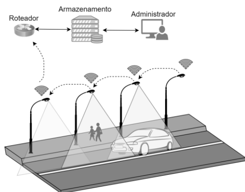
Figura 1. Representação de RSSF para sistemas de iluminação pública.
