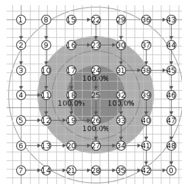
Figura 5. Exemplo de cenário de rede com 48 sensores e um coordenador no simulador Cooja.
