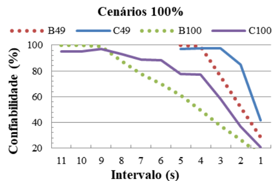
Figura 6. Confiabilidade dos protocolos em cenários com 100% de garantia de entrega ponto-a-ponto.
