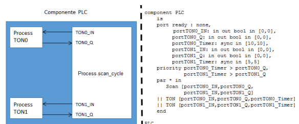
Figura 4: Component PLC em FIACRE do programa em LD ilustrado na Figura 3
