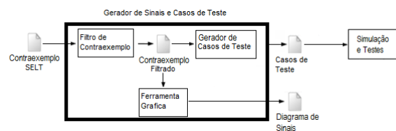
Figura 9: Processo de tradução do contraexemplo
