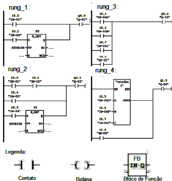
Figura 3: Exemplo de programa em LD
