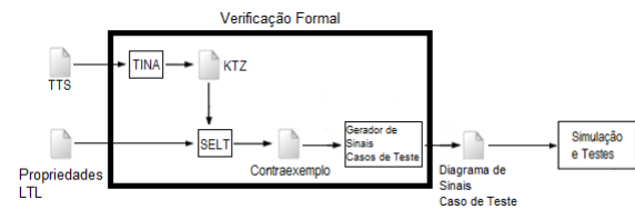
Figura 8: Etapa de Verificação Formal
