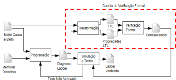
Figura 1: Metodologia de verificação formal proposta
