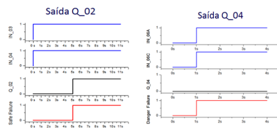
Figura 10: Contraexemplo na forma de diagrama de sinais para os efeitos Q_02 e Q_04
