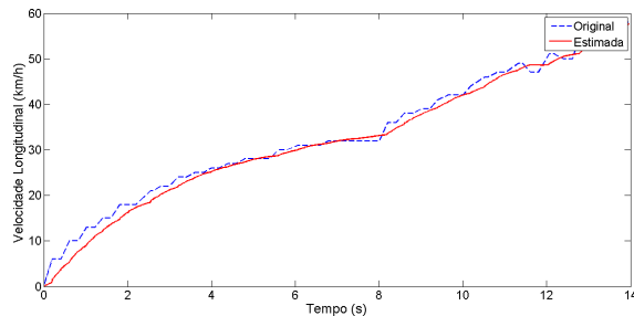
Figura 4: Velocidade longitudinal estimada pelo filtro de Kalman.
