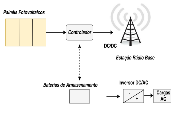
Figura 1: Configuração típica de uma Estação Rádio Base alimentada por painéis fotovoltaicos.
