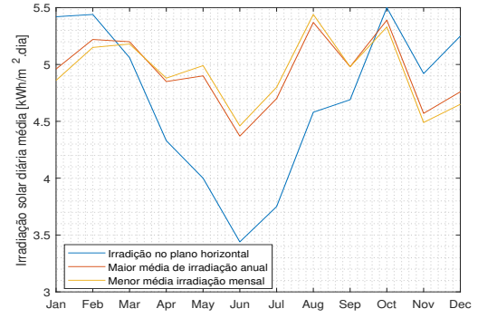
Figura 2: Perfil de irradiação diária média na cidade de Santa Rita do Sapucaí - MG.
