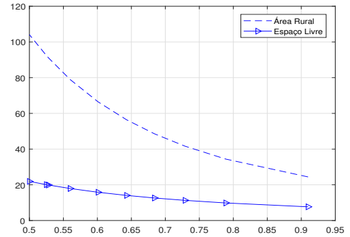
Figura 3: Influência do ambiente no consumo de potência de uma ERB.
