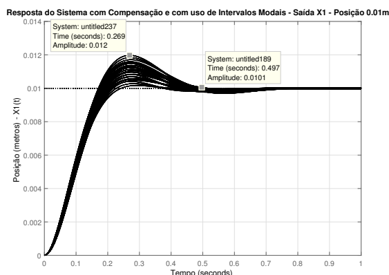
Figura 8: Resposta da Saída x_1 do Sistema Compensado com o uso de Intervalos Modais para a Posição 0,01m e com os valores de ganhos do Compensador Convencional.
