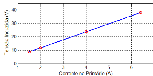
Figura 8. Tensão Induzida x Corrente no Primário.
