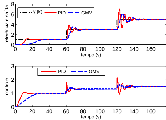
Figura 4: Resposta do sistema com os controladores PID e GMV.
