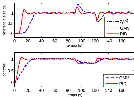
Figura 7: Resposta do sistema com sinal de ruído e perturbação - controladores PID e GMV.
