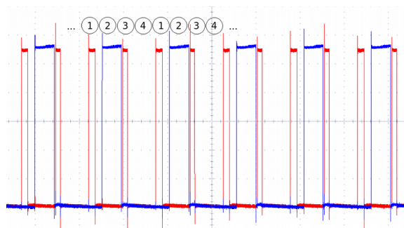
Figura 4. Visualização das trocas de contexto e da tarefa Idle .
