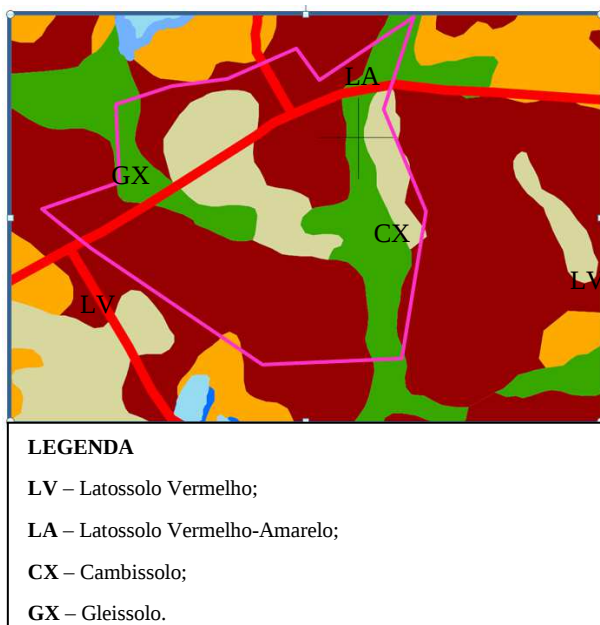
Figura 3 – Grupos de solos da região (Modificado - EMBRAPA, 2004).
