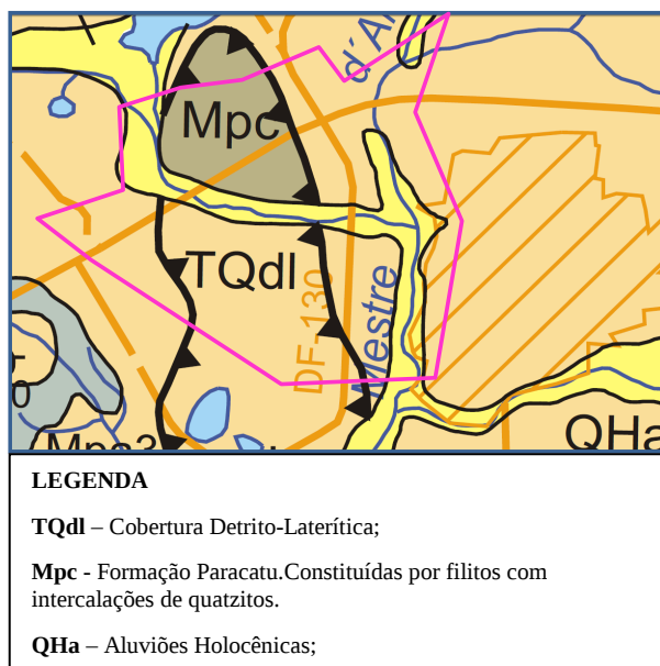
Figura 4 - Formação Geológica da região (Modificado - ZEE (2002).
