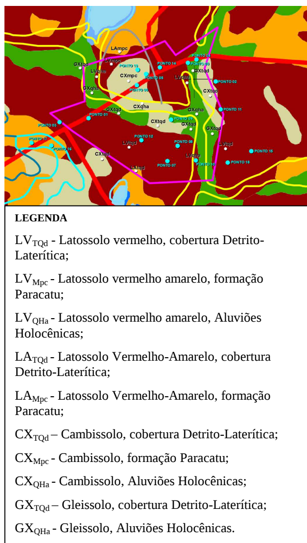
Figura 5 - Unidades Geotécnicas da região e localização dos pontos estudados.
