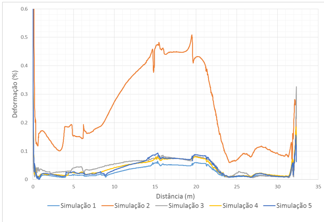
Figura 3. Deformação da geomembrana.
