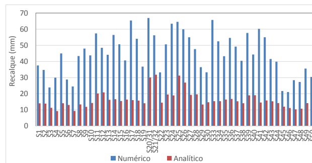
Figura 8. Recalque previsto pelo método numérico e recalque calculado pelo método analítico
