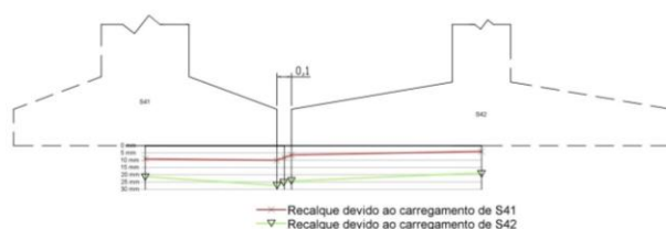
Figura 12. Recalque causado pela influência entre as sapatas S41 e S42.
