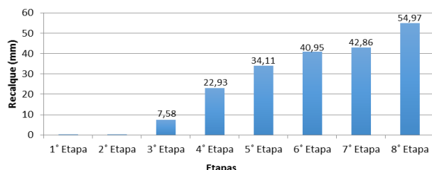
Figura 14. Recalque acumulado por etapa na sapata S42.
