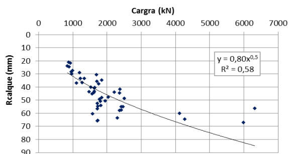
Figura 10. Carga versus recalque numérico
