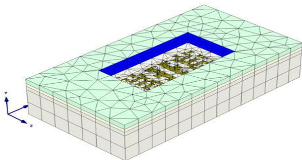
Figura 6. Modelagem do terreno escavado, com contenção e com fundação.
