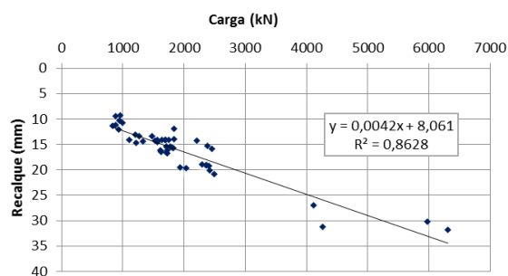
Figura 9. Carga versus recalque analítico.
