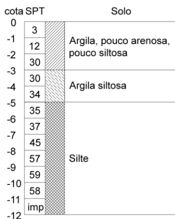
Figura 4. Perfil de solo do local da obra.
