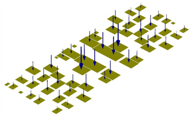
Figura 7. Vista isométrica das sapatas com seus vetores de cargas correspondentes.
