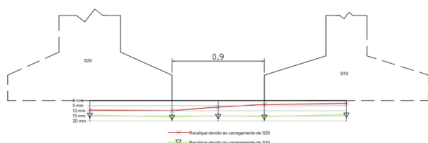
Figura 11. Recalque causado pela influência entre as sapatas S29 e S19.
