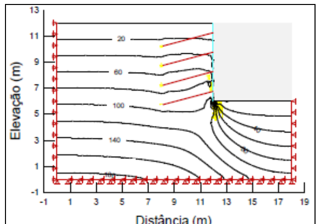
Figura 15. Zonas de plastificação.
