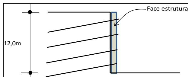
Figura 20. Tirantes com face estruturada.
