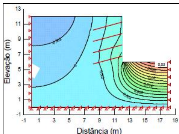
Figura 12. Deslocamentos verticais - recalques.
