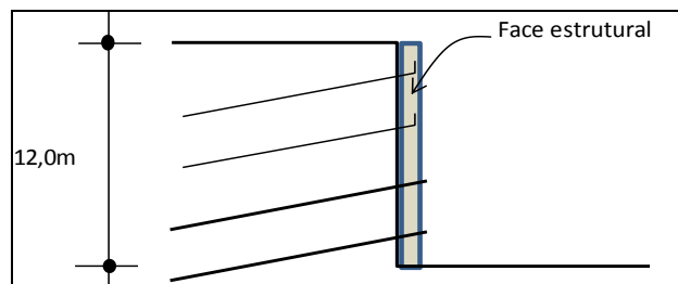
Figura 21. Estrutura mista - grampos e tirantes com face em concreto estrutural (Caso 2C).
