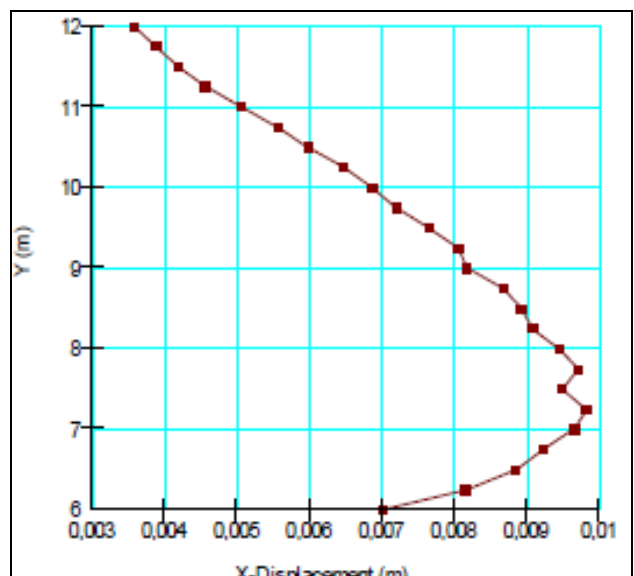
Figura 16. Gráfico dos deslocamentos horizontais da face.
