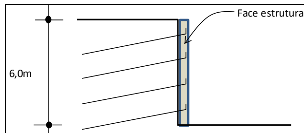
Figura 19. Solo grampeado com parede estrutural (Caso 2A).
