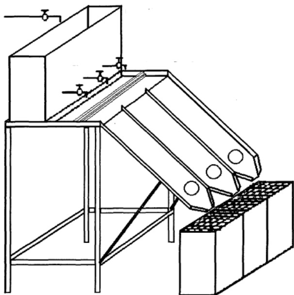
Figura 3. Modelo de aparelho proposto por Fácio (1991). Adaptado de Fácio (1981 apud LEMOS, 2002)
