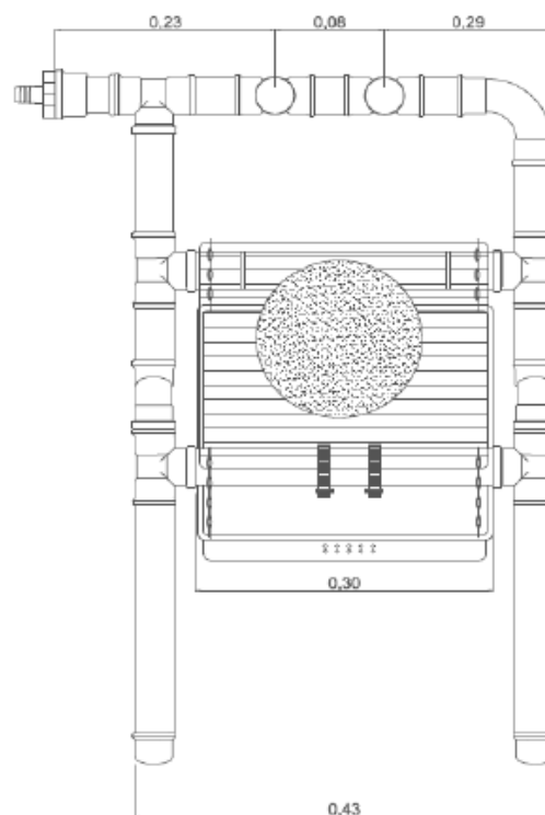
Figura 6. Modelo de aparelho proposto por Quirino; Moraes; Melo (2013). Adaptado de QUIRINO; MORAIS; MELO (2013).
