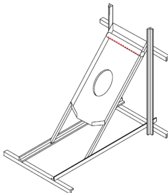
Figura 2. Modelo de aparelho proposto por Fonseca e Ferreira (1981). Adaptado de Fonseca e Ferreira (1981 apud LEMOS, 2002)
