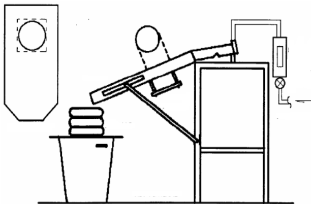
Figura 4. Modelo de aparelho proposto por Bastos (1999). Adaptado de Bastos (1999 apud LEMOS, 2002)
