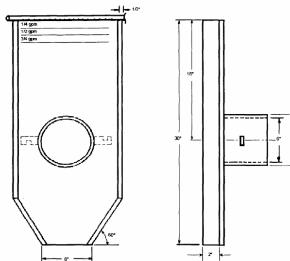
Figura 1. Modelo de aparelho proposto por Inderbitzen (1961). Adaptado de Inderbitzen (1961 apud LEMOS, 2002)
