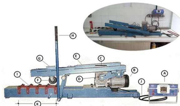
Figura 3. Equipamento LWT - detalhes.
