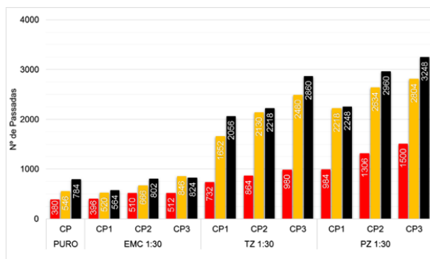
Figura 6. Resultados dos Ensaios LWT utilizando a dosagem 1:30
