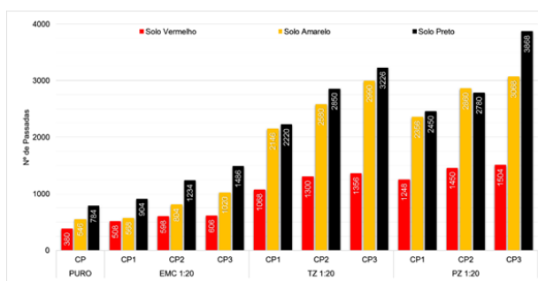
Figura 7. Resultados dos Ensaios LWT utilizando a dosagem 1:20
