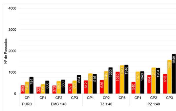
Figura 5. Resultados dos Ensaios LWT utilizando a dosagem 1:40
